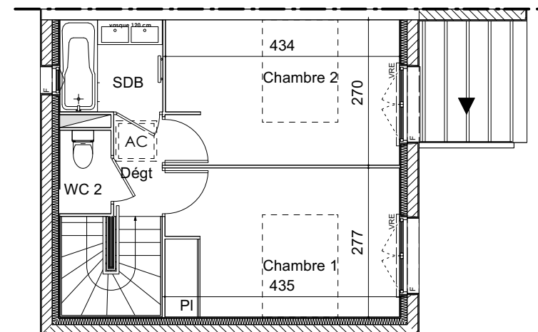
PLAN ETAGE
