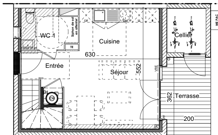
PLAN REZ-DE-CHASSE
