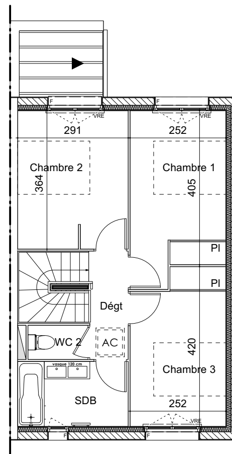
PLAN ETAGE
